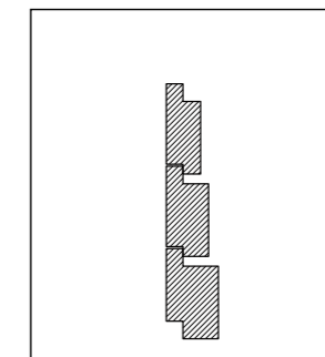
Deckleist Stufenfalz 3D
