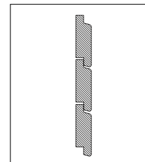
Falzprofil mit schräger Kante
